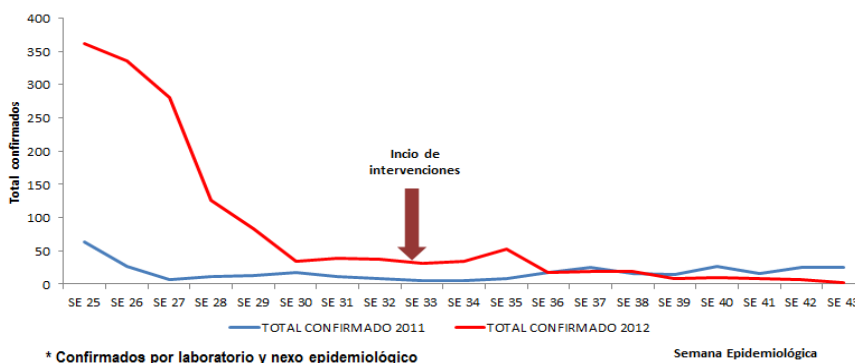
Comparativo de casos confirmados* de Dengue, según semana epidemiológica. Año 2011 y 2012. Periodo: SE 25 a 43.
