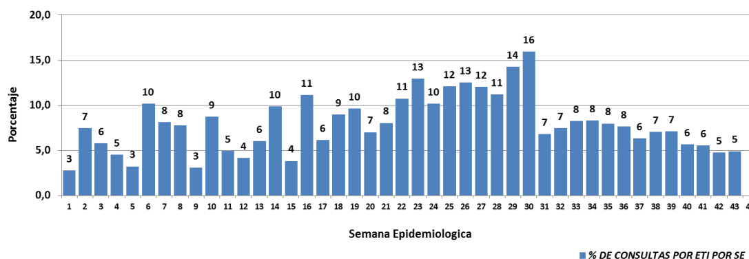
Proporción de consultas por ETI según semana epidemiológica del 1 al 43 Paraguay, 2012
