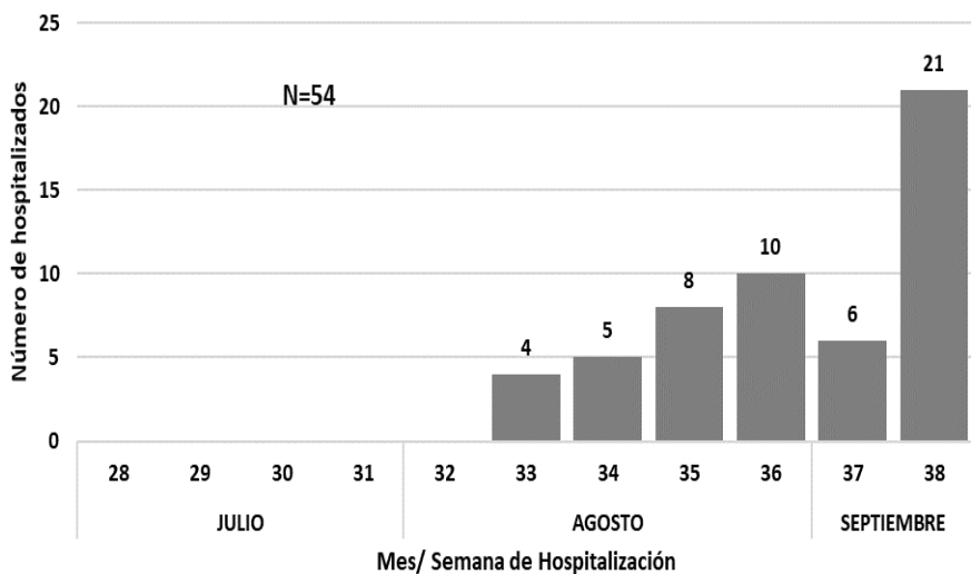
Distribución por semana de hospitalización. Casos confirmados COVID-19, hospitalizados entre las SE 28 y 38 (julio a septiembre parcial). Año 2020 CORDILLERA
