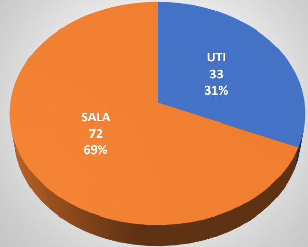
Sitio de hospitalización n=105
