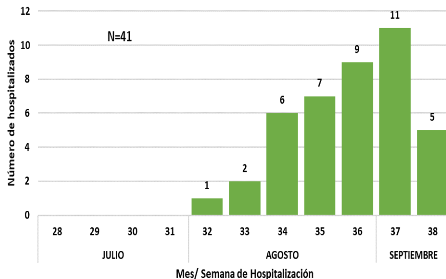
Distribución por semana de hospitalización. Casos confirmados COVID-19, hospitalizados entre las SE 28 y 38 (julio a septiembre parcial). Año 2020 ITAPÚA
