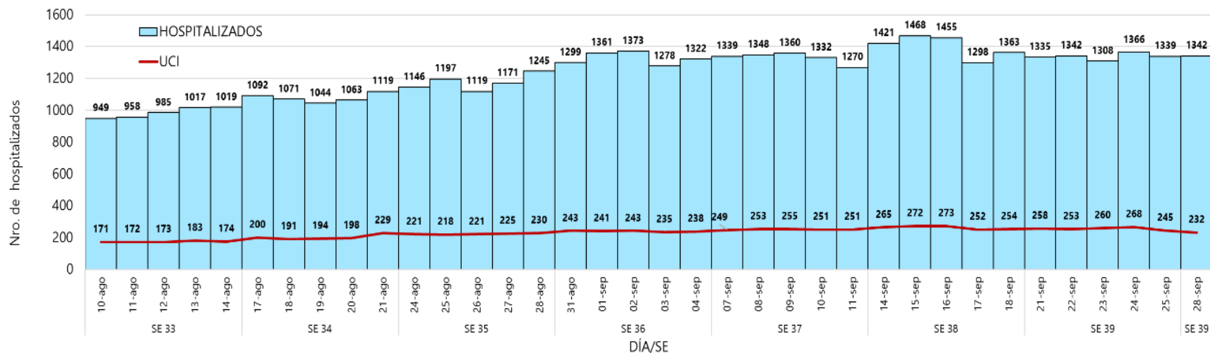
Hospitalizados acumulados UCI /RAG, desde la SE 33 (10 08) a SE 40 (28 09) Año 2020
