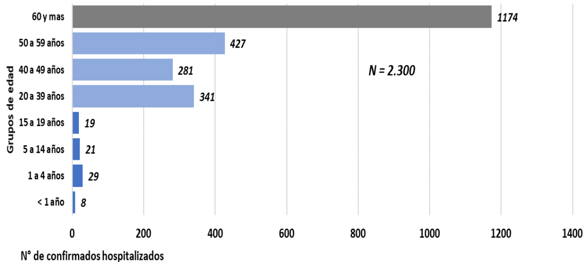
Número total de casos confirmados COVID-19, según grupos de edad, hospitalizados entre las SE 28 y 38 (julio a septiembre parcial), Paraguay - 2020
