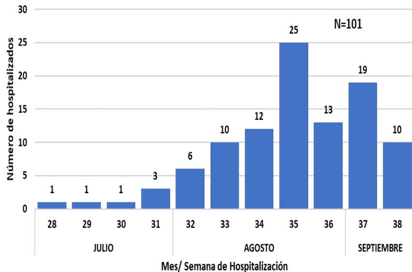
Distribución por semana de hospitalización. Casos confirmados COVID-19, hospitalizados entre las SE 28 y 38 (julio a septiembre parcial). Año 2020 CAAGUAZU
