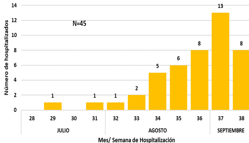
Distribución por semana de hospitalización. Casos confirmados COVID-19, hospitalizados entre las SE 28 y 38 (julio a septiembre parcial). Año 2020 GUAIRÁ
