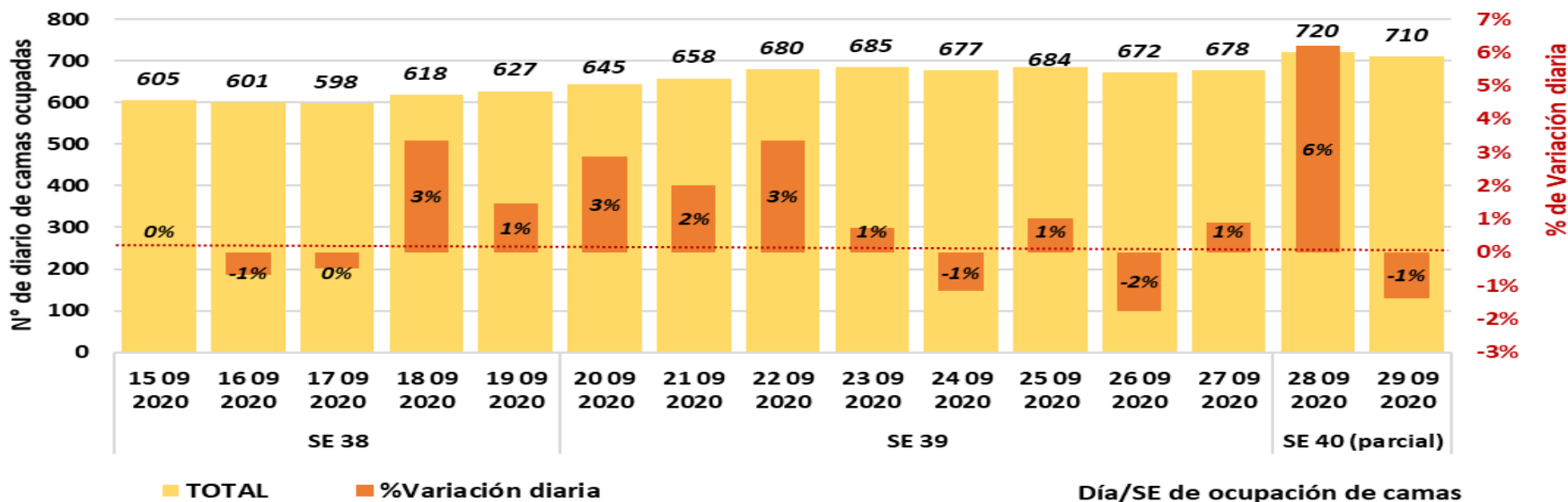
Número diario de camas ocupadas por hospitalizados confirmados COVID-19, y porcentaje de variación diaria.
