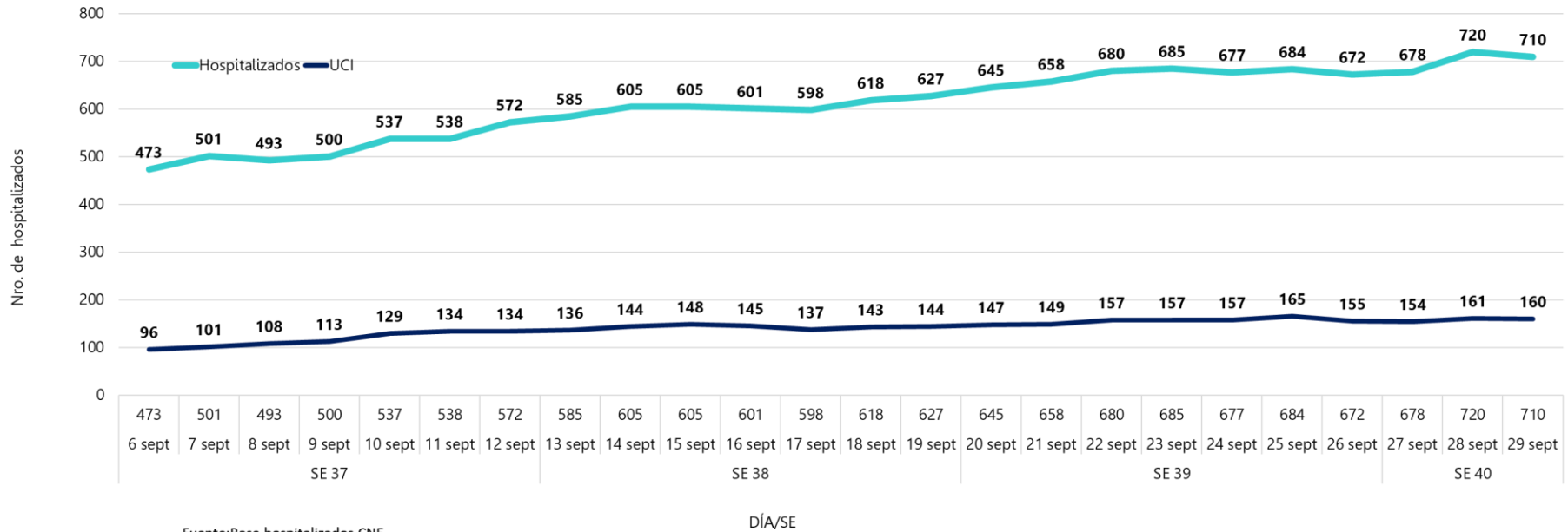
Hospitalizados por COVID-19 desde la SE 37 (06 09) a SE 40 (29 09) Año 2020
