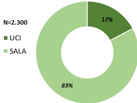
Distribución porcentual de hospitalizados confirmados para COVID-19, según condición de ocupación de servicio de Sala o UCI
