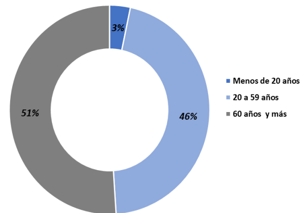
Distribución porcentual según grupos de edad. Casos confirmados COVID-19, hospitalizados entre las SE 28 y 38 (julio a septiembre parcial), Paraguay - 2020
