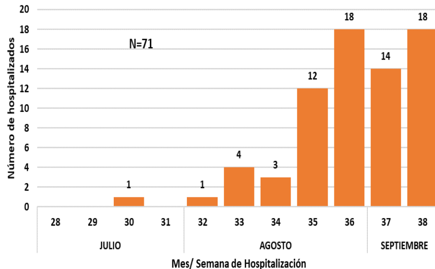
Distribución por semana de hospitalización. Casos confirmados COVID-19, hospitalizados entre las SE 28 y 38 (julio a septiembre parcial). Año 2020 CONCEPCIÓN
