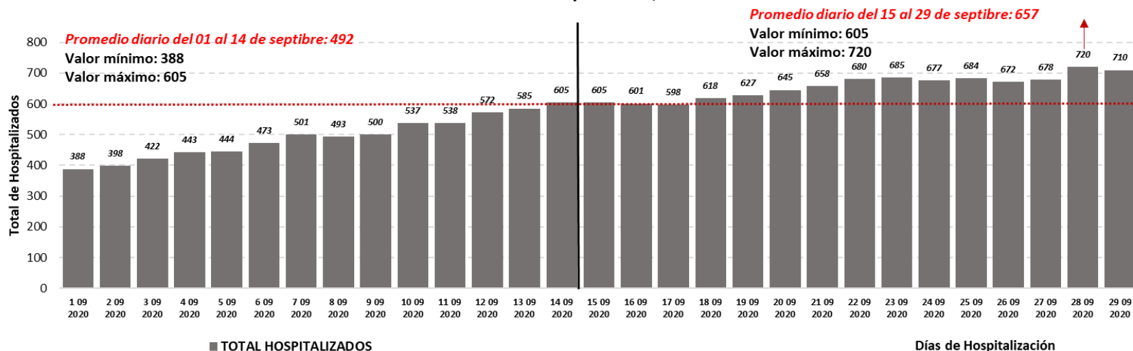
Número diario de hospitalizados casos confirmados COVID-19, en todo el país. Periodo: 01 al 29 de septiembre, año 2020
