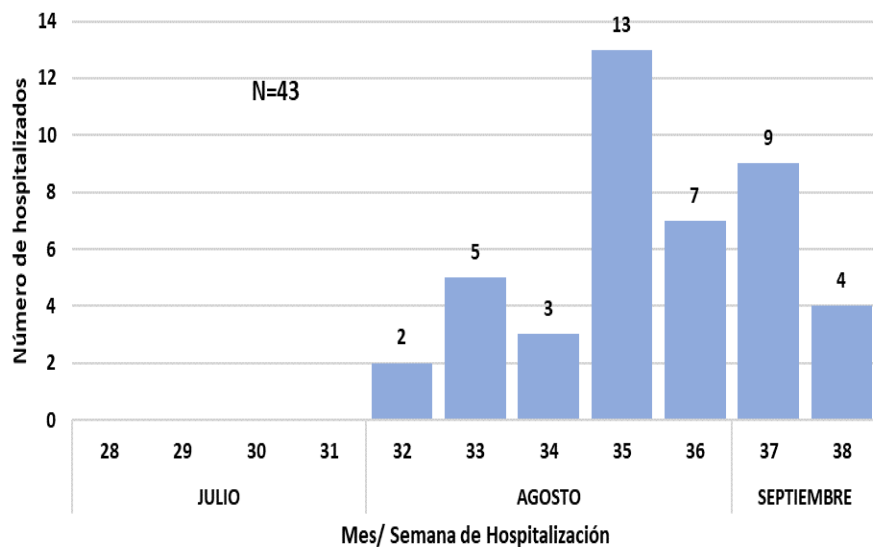
Distribución por semana de hospitalización. Casos confirmados COVID-19, hospitalizados entre las SE 28 y 38 (julio a septiembre parcial). Año 2020 AMAMBAY
