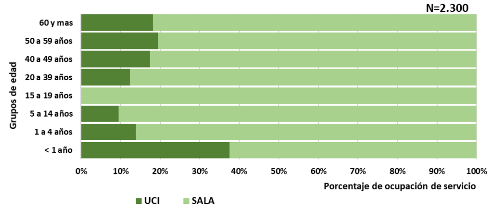
Distribución porcentual de hospitalizados confirmados para COVID-19, según grupos de edad y condición de ocupación de servicio de Sala o UCI
