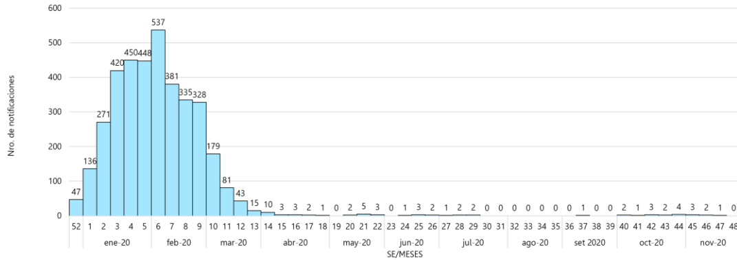
Notificaciones de dengue. SE1 a SE 48. Departamento Cordillera. Año 2020
