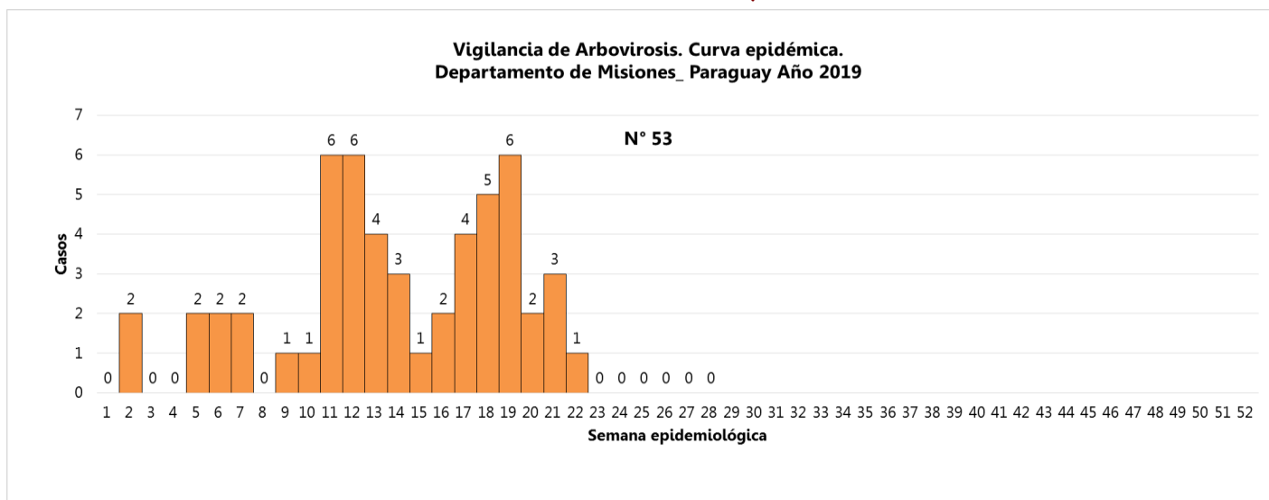
Gráfico 1: Curva de notificaciones, Misiones. (Probables y Sospechosos)- SE 1 a la SE 28. Año 2019
