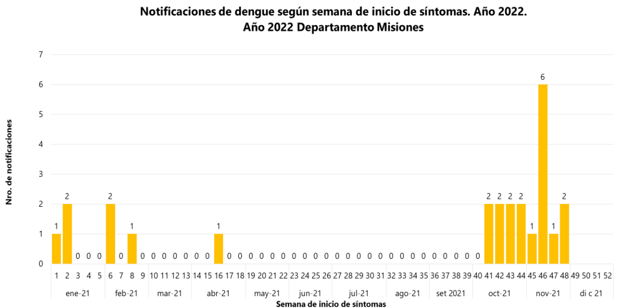
Gráfico 1. Dengue. Número de notificaciones desde la SE 1 a la SE 48, departamento de Misiones, año 2022
