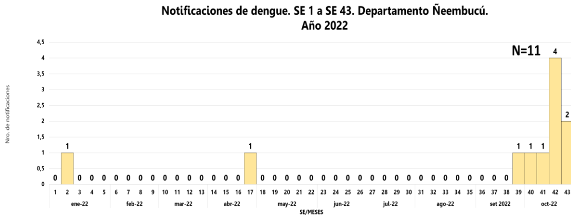
Gráfico 1. Dengue. Número de notificaciones desde la SE 1 a la SE 43, departamento de Ñeembucú, año 2022
