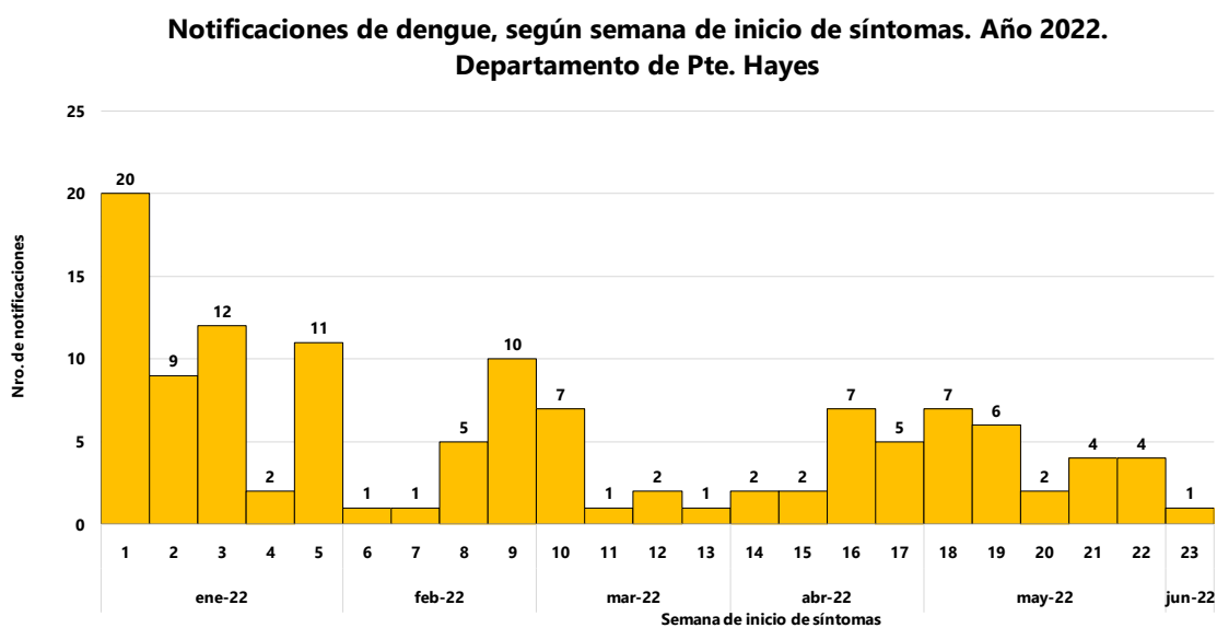
Gráfico 1. Dengue. Número de notificaciones desde la SE 1 a la SE 23, departamento de Pte. Hayes, año 2022
