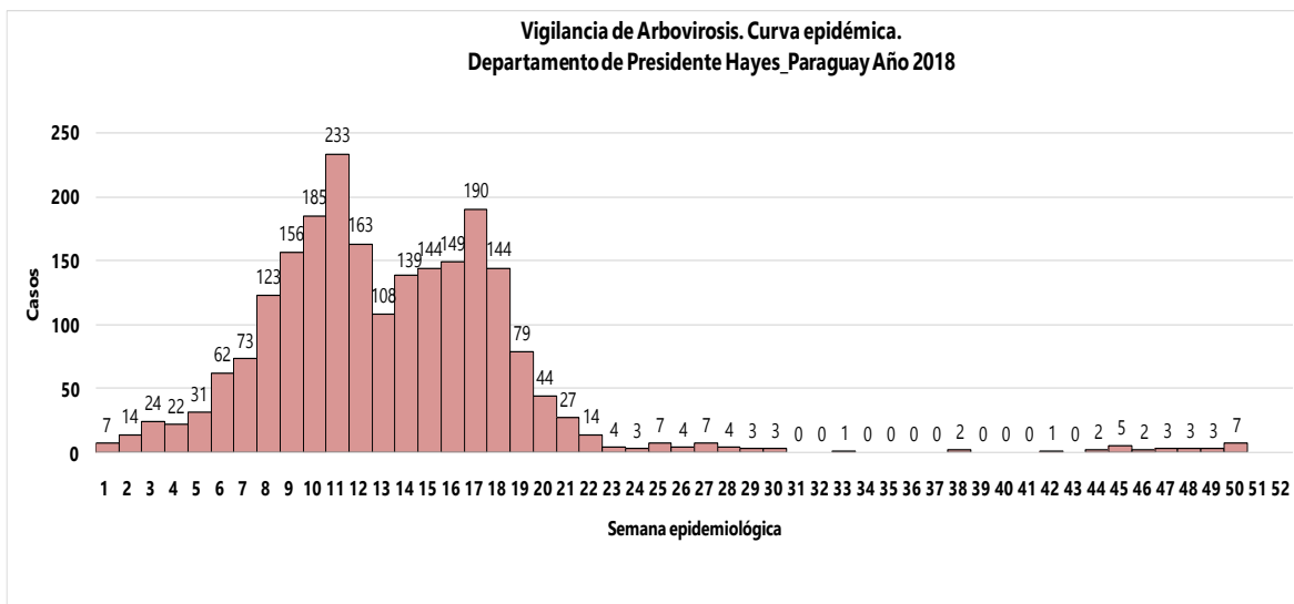
Gráfico1: Curva de notificaciones Pte. Hayes-SE 1 a la SE 50. Año 2018
