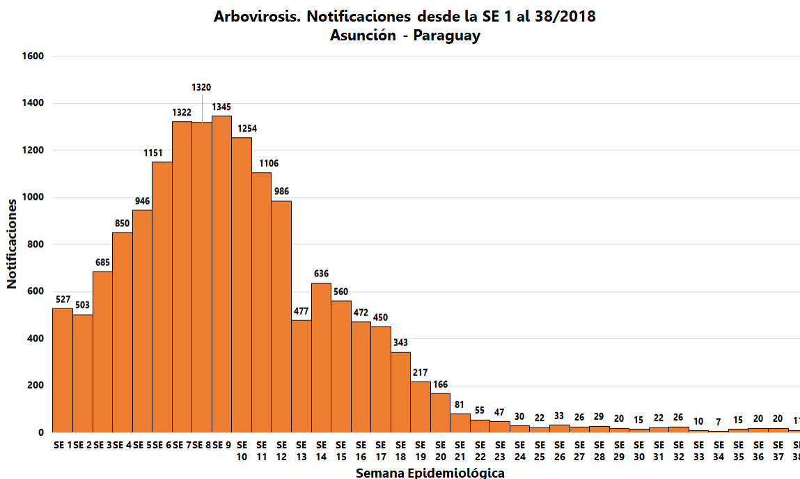
Gráfico 1: Curva de notificaciones, Asunción-SE 1 a la SE 38. Año 2018
