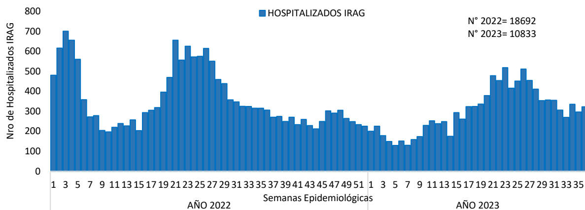
Gráfico 11. Número de hospitalizados por IRAG según semana epidemiológica, Vigilancia Centinela, Paraguay, SE 1 del 2022 a SE 36 del 2023.
