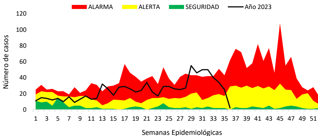
Gráfico 27. Canal endémico de varicela según semana de inicio de síntomas, Paraguay, SE 1 a la SE 36 del 2023.
