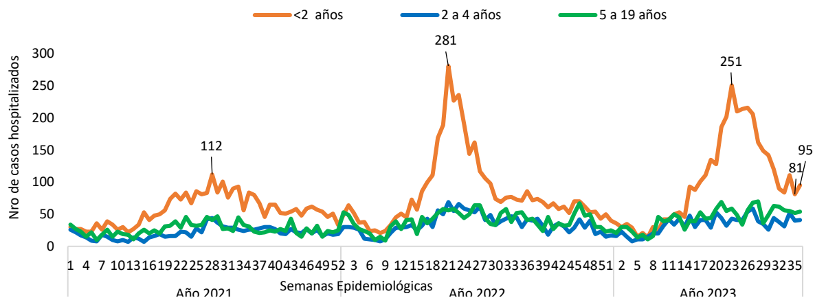
Gráfico 12. Casos hospitalizados por IRAG en edad pediátrica según semana epidemiológica, Vigilancia Centinela, Paraguay, años 2021, 2022 y 2023 (hasta la SE 36).
