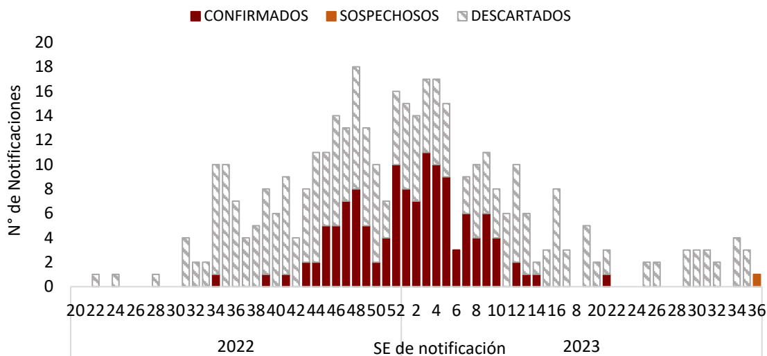
Gráfico 28. Curva de notificaciones de Viruela Símica según clasificación final y semana de notificación, Paraguay, desde SE 21 del 2022 a SE 36 del 2023.
