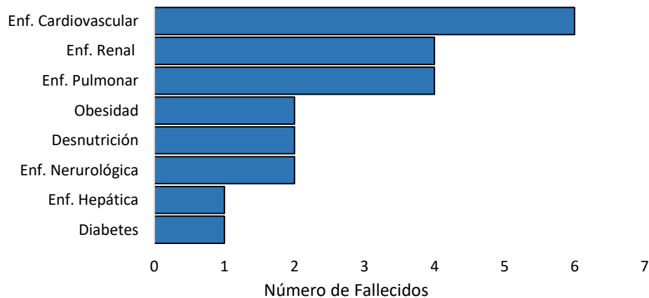
Gráfico 7. Comorbilidades de los fallecidos confirmados por COVID-19, Paraguay, desde la SE 29 a la SE 36 del 2023.
