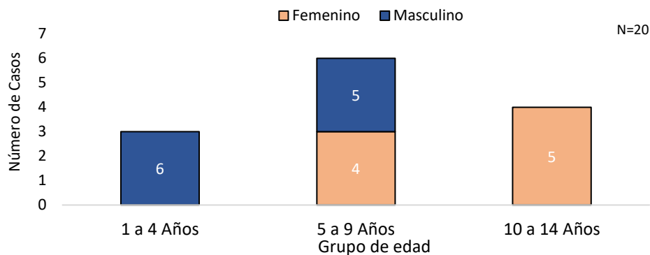
Gráfico 26. Número de casos de PFA según grupo de edad y sexo, Paraguay, SE 1 a la SE 36 del 2023.
