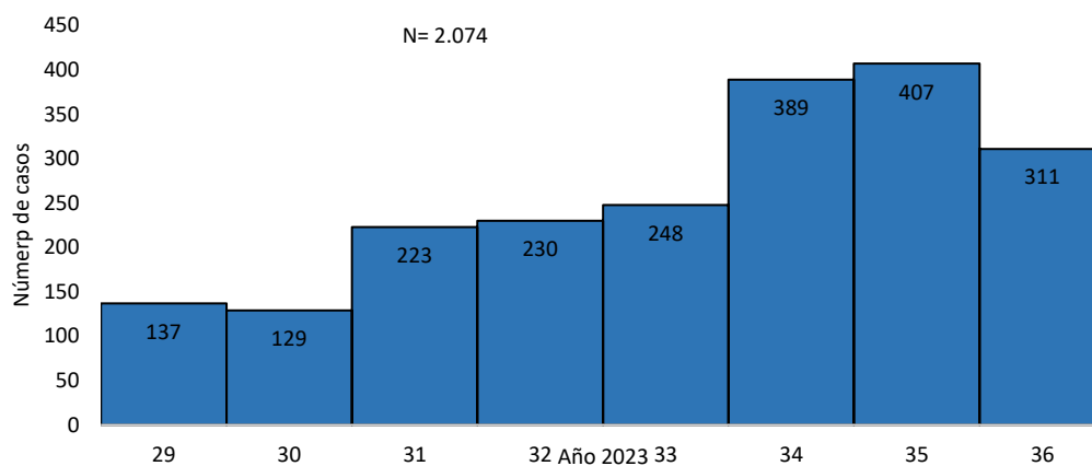
Gráfico 4. Curva epidémica de casos COVID-19, según semana epidemiológica, Paraguay, SE 29 a SE 36 del 2023.
