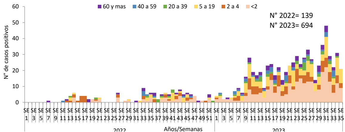
Gráfico 17. Distribución de casos hospitalizados IRAG positivos según grupos de edad. Vigilancia Centinela, Año 2022(SE 1-52) y 2023 (SE 1-36).
