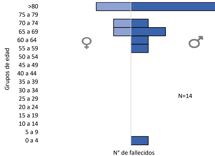
Gráfico 6. Fallecidos confirmados por COVID-19, por grupos de edad y sexo edad, Paraguay, desde la SE 29 a la SE 36 del 2023.
