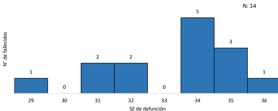
Gráfico 5. Fallecidos confirmados por COVID-19, según semana de defunción, Paraguay, SE 29 a SE 36 del 2023.
