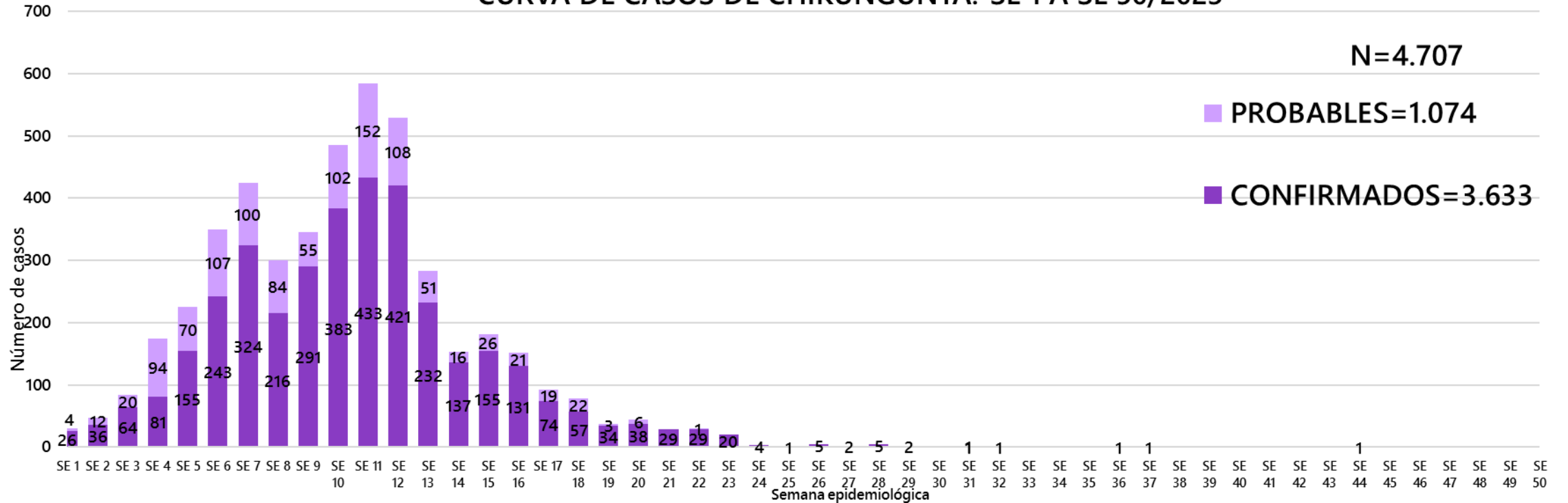
CURVA DE CASOS DE CHIKUNGUNYA. SE 1 A SE 50/2023
