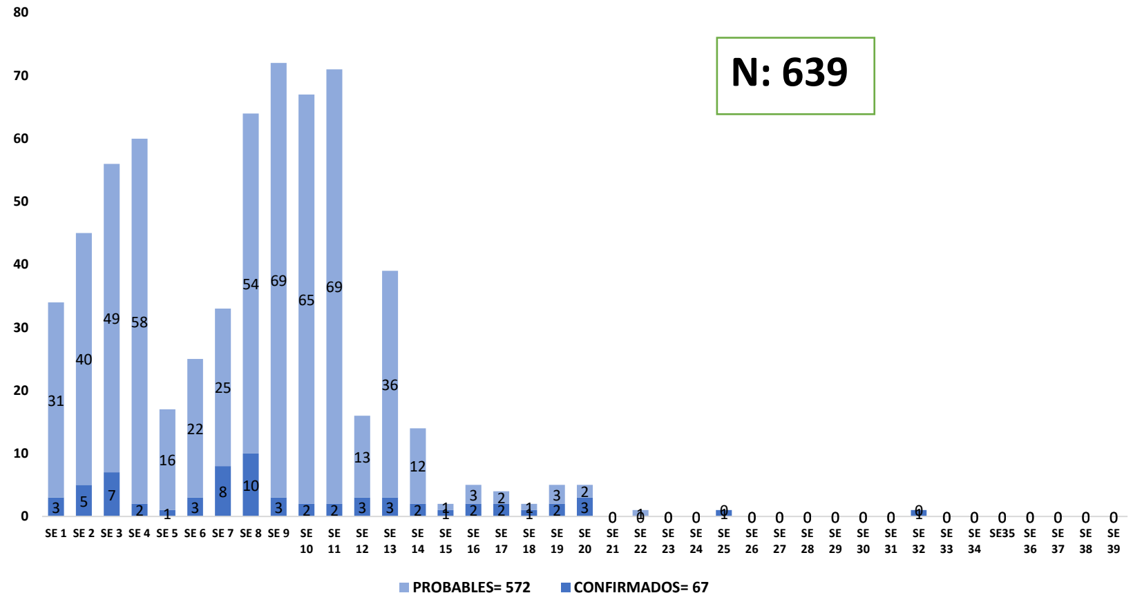
CURVA DE CASOS DE DENGUE. SE 1 A SE 39/2024
